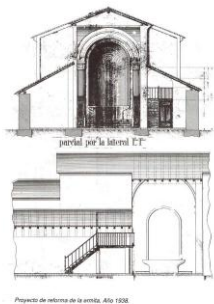
Planos de la ermita construida en 1939.
