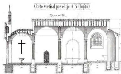
Planos de la ermita construida en 1939.
